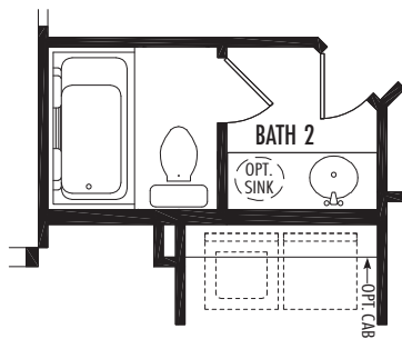
OPTIONAL BATH 2
