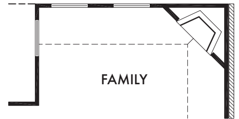
OPTIONAL FIREPLACE OPT. #300
