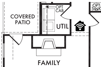
OPTIONAL FIREPLACE
