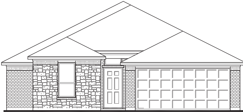
ELEVATION I
