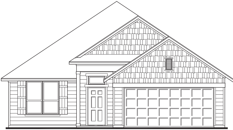
ELEVATION A
