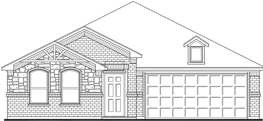
ELEVATION J
